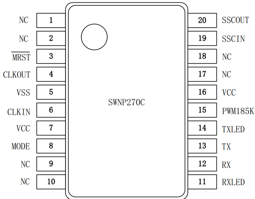
图2 引脚图
