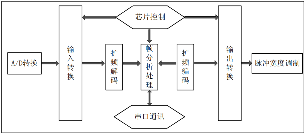
图1 功能方框图
