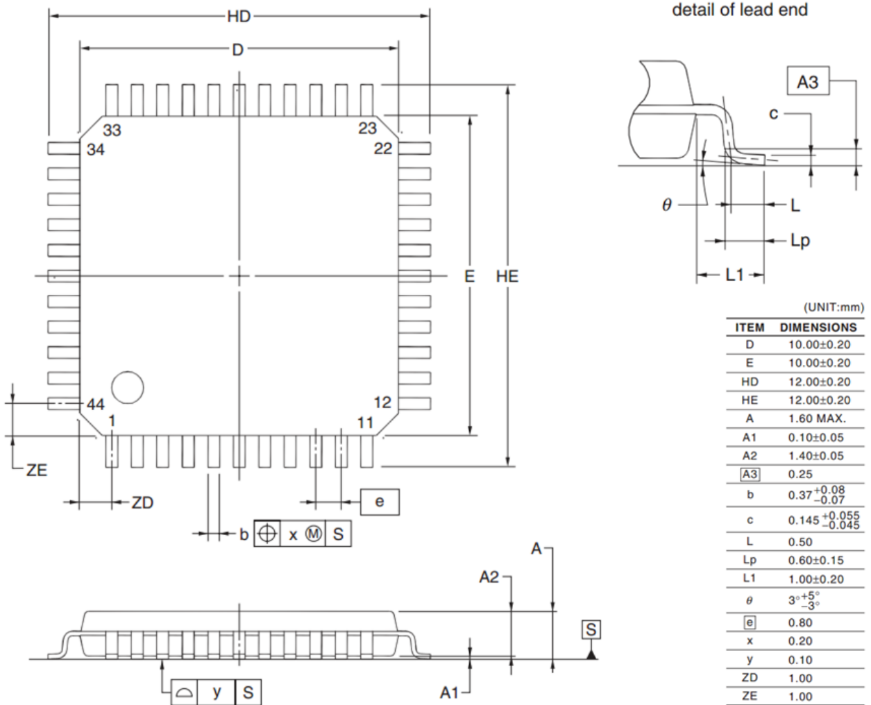
图 3 封装图
