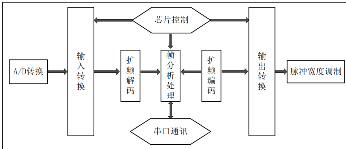
图 1 功能方框图
