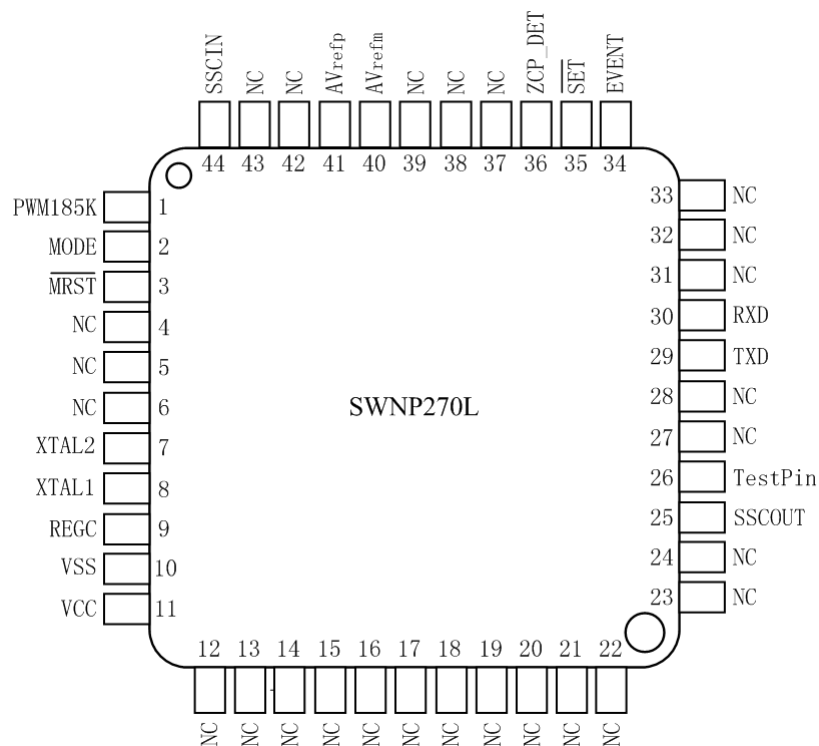
图 2 引脚图
