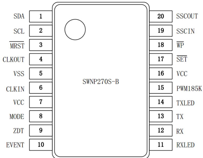
图 2 引脚图
