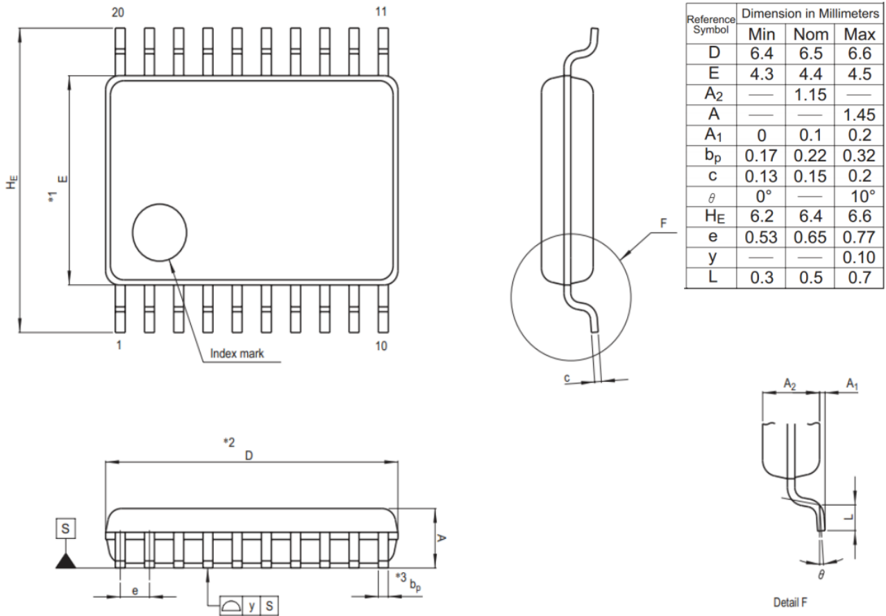
图 3 封装图
