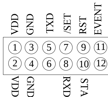
图 4 SWMW470T 模块引脚定义图
