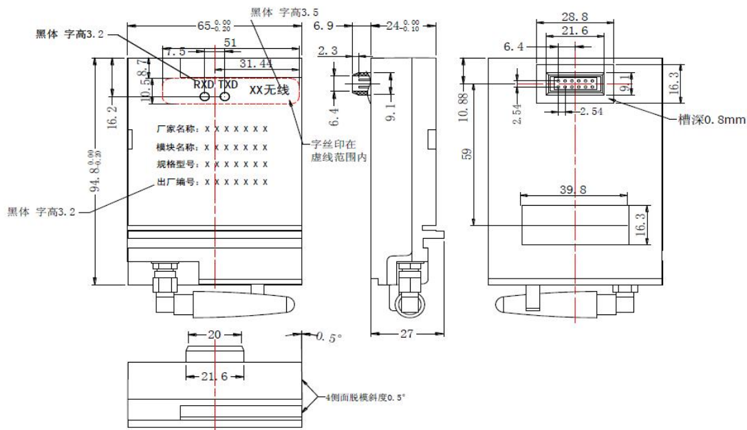
图 7 模块正视、侧视、底视示意图
