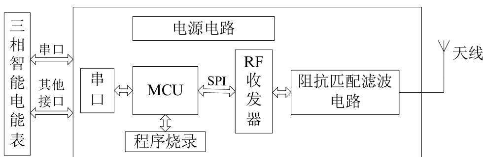
图2 三相表无线模块工作原理框图
