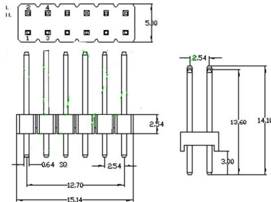
图 8 2×6 双排插针
