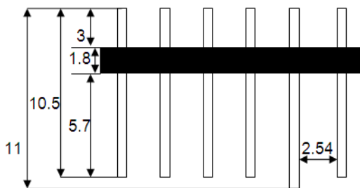
图 7 2×6 双排插针
