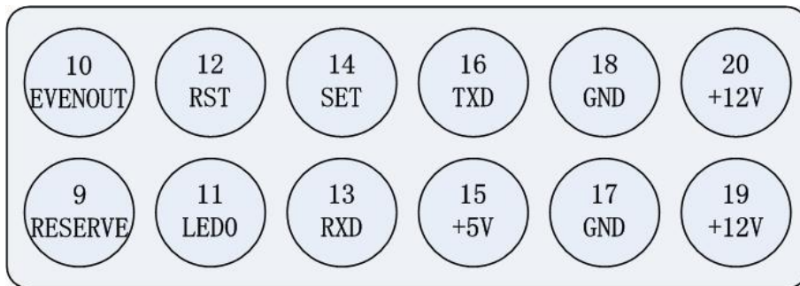
图 4 模块弱电接口示意图
