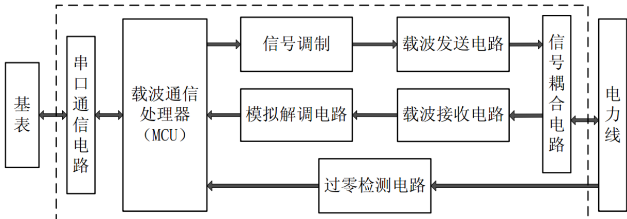
图2 载波工作原理框图
