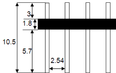
图 8 2×4 双排插针
