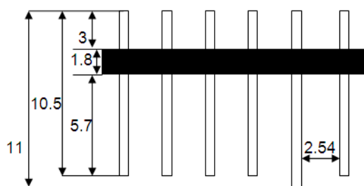
图 7 2×6 双排插针
