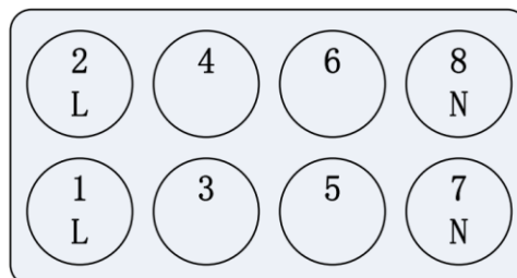
图 5 模块载波耦合接口示意图
