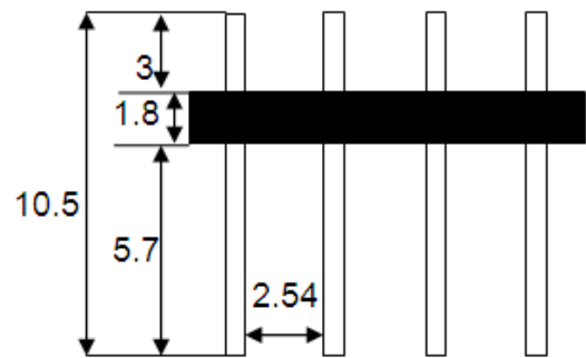
图 8 2×4 双排插针
