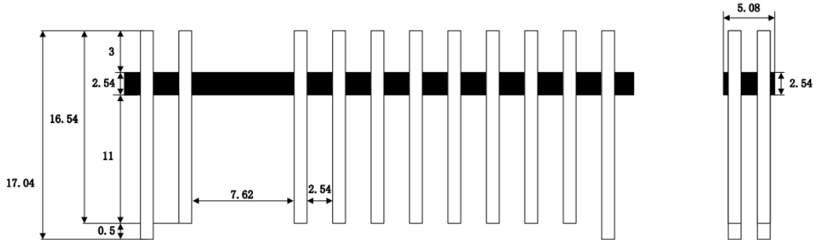
图 7 2×11 双排插针
