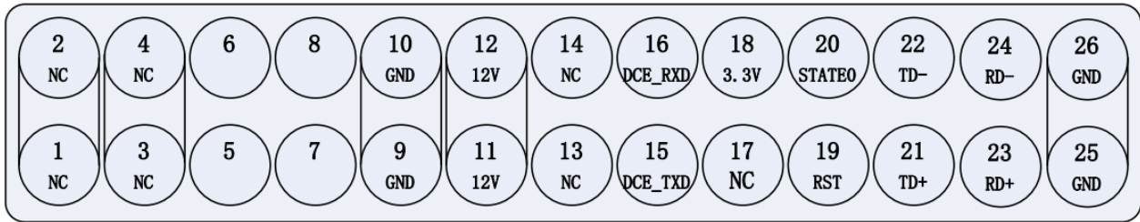
图 4 本地通信模块接口定义
