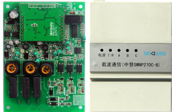
图 1 集中器载波模块和外壳
