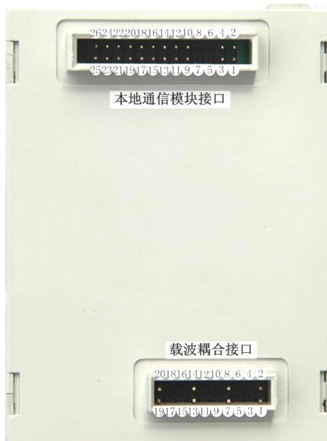
图3 模块接口底视图
