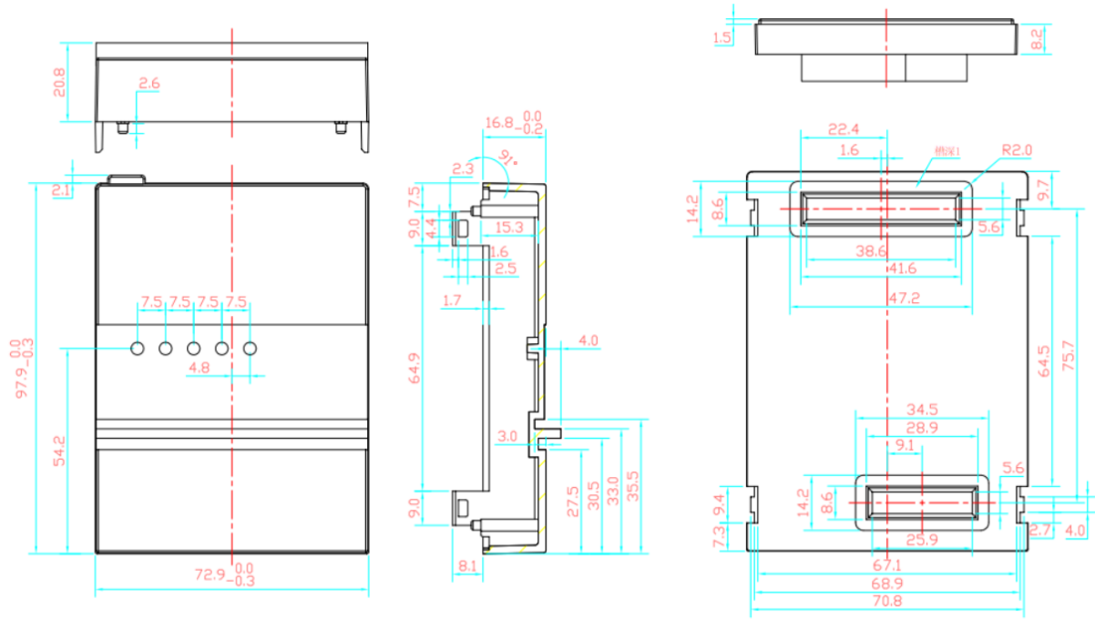
图 6 模块正视、侧视、底视尺寸图
