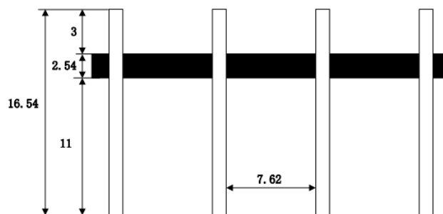
图 8 2×4 双排插针
