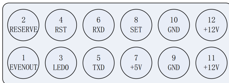
图 4 模块弱电接口示意图
