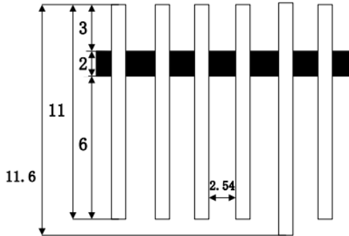
图 7 2×6 双排插针
