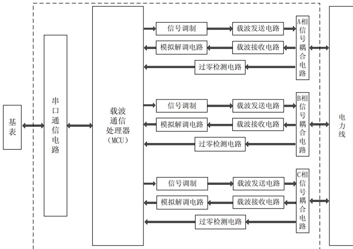
图2 工作原理框图
