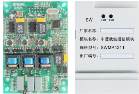
图 1 三相载波通信模块
