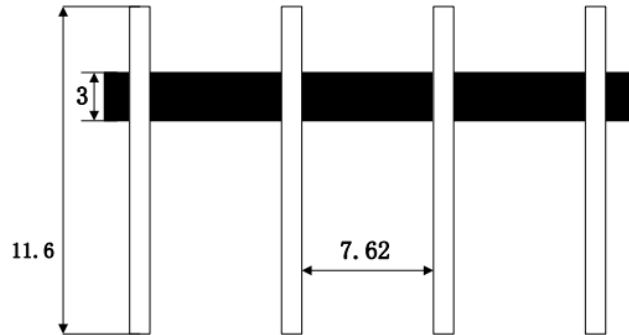
图 8 2×4 双排插针
