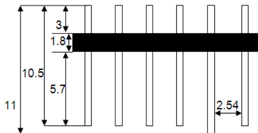
图 7 2×6 双排插针
