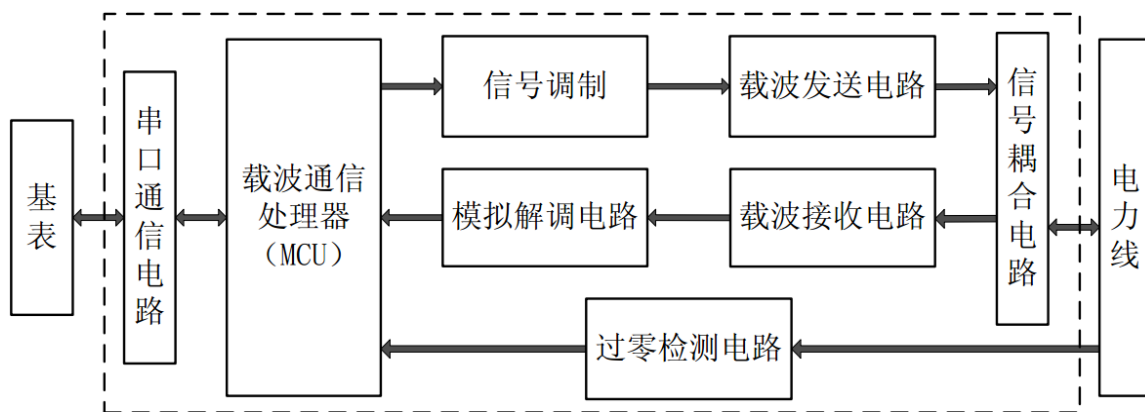
图2 载波工作原理框图
