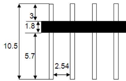
图 8 2×4 双排插针
